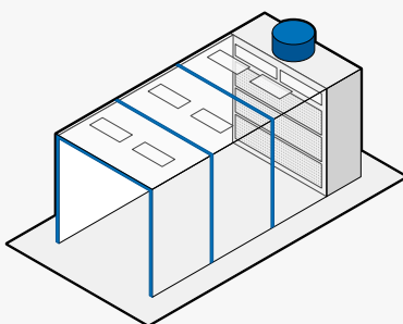
➤ Cabina di verniciatura con avancorpo con pareti e tetto in pannelli precoibentati verniciati e luci
