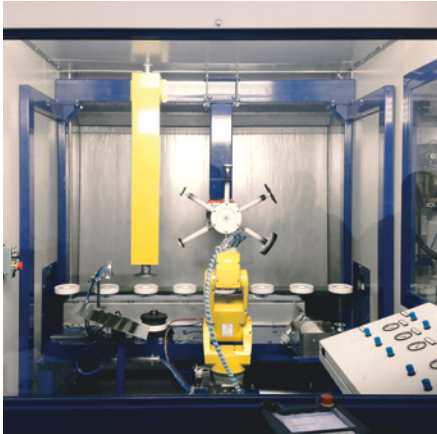
➤ Cabine di verniciatura a velo d'acqua
