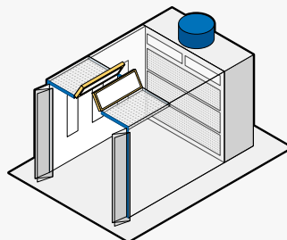
➤ Cabina di verniciatura flusso obliquo con entrata aria a tetto filtrata e portone a libro
