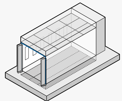
➤ Cabina di verniciatura pressurizzata con plenum di immissione aria filtrato e aspirazione a pavimento
