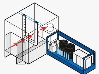
➤ Skid 5 stadi con portale per lavaggio automatico per lavare in automatico e in manuale nella stessa cabina
