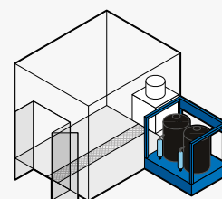
➤ Skid 2 stadi Sgrassaggio + risciacquo
