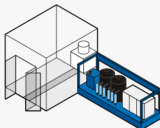
➤ Skid 4 stadi Sgrassaggio a caldo, 2 risciacqui + risciacquo osmo
