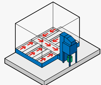
➤ Recupero automatico sopra pavimento senza fondazione, con piano di lavoro sopraelevato
