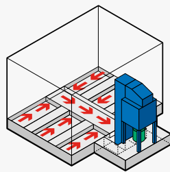
➤ Recupero automatico con fondazione completa
