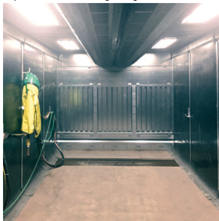
➤ Cabine di granigliatura con recupero parziale della graniglia
