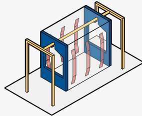
➤ Tunnels IR avec panneaux à infrarouges
