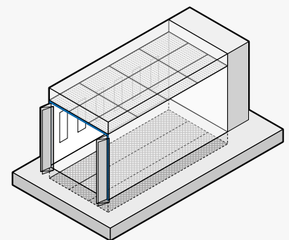
➤ Überdrucklackierkabine mit gefilterter Luftzufuhr über Filterplenum in Decke und Bodenabsaugung
