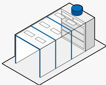
➤ Lackierkabinen mit Gehäuse mit isolierten Paneelwänden, Decke und Beleuchtung
