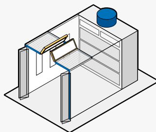
➤ Lackierkabinen mit vertikalem Luftstrom mit gefilterter Luftzufuhr über Kabinendach und Falttor
