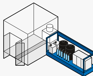
➤ Skid 5 étages Dégraissage à chaud, 2 rinçages + rinçage osmo + passivant
