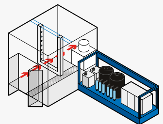
➤ Skid 5 étages avec portique de lavage automatique pour laver en mode automatique et manuel dans la même cabine
