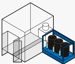
➤ Skid 3 étages Solution standard: dégraissage + 2 rinçages
