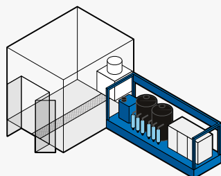
➤ Skid 4 Phasen Heißentfettung, 2 Spülungen + VE-Spüle
