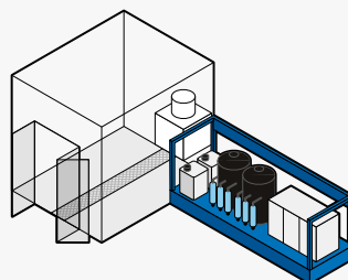
➤ Skid 5 Phasen Heißentfettung, 2 Spülungen, VE-Spüle + Passivierung
