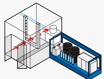
➤ Skid 5 Phasen mit automatischem Waschportal für automatisches und manuelles Waschen in einer Kabine
