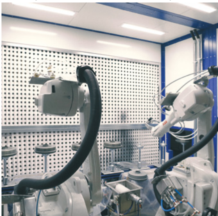
➤ Impianti di verniciatura a liquido automatici in continuo con convogliatore rovesciato
