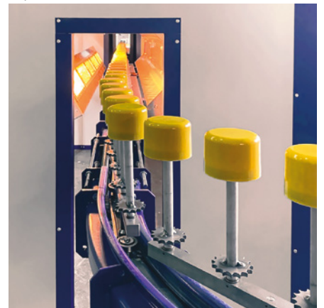
➤ Impianto di verniciatura a liquido automatico passo-passo con convogliatore rovesciato per automotive
