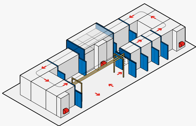
➤ Impianto di verniciatura a liquido passo-passo
